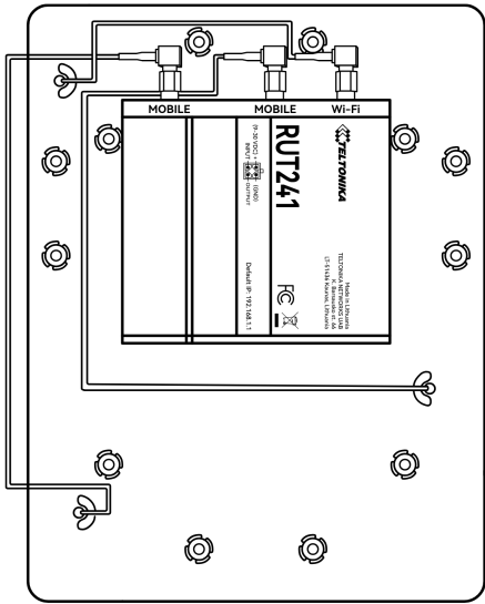
TELTONIKA RUT241
